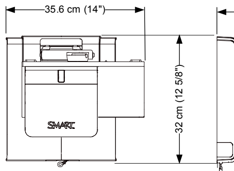
Интерактивный проектор, вид спереди
