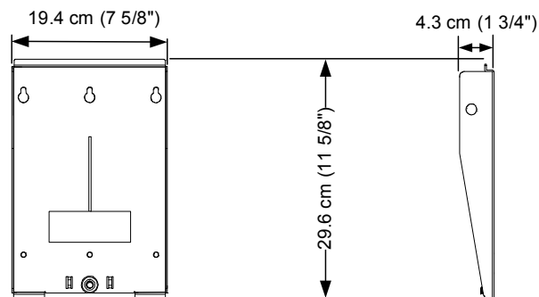
Монтажная планка, вид спереди
