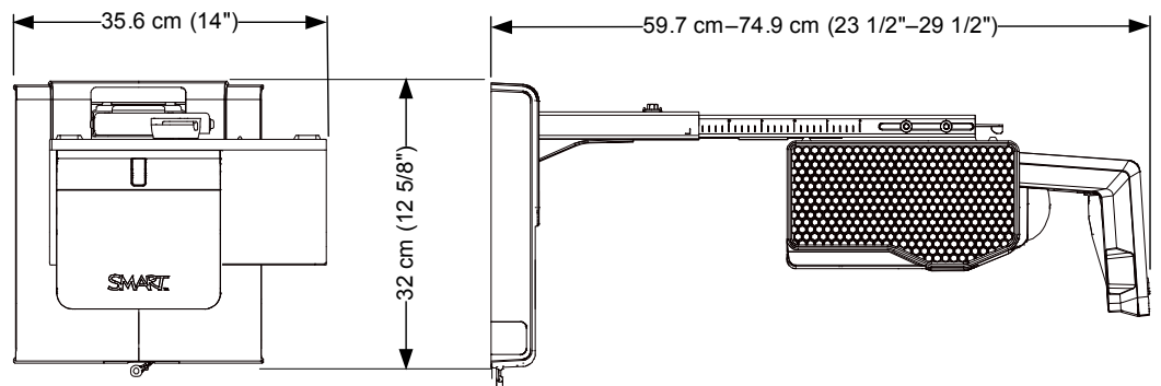
Интерактивный проектор, вид спереди
